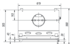
Wkład kominkowy ZUZIA 16 kW z wermikulitem
