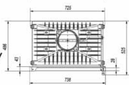
Wkład kominkowy OLIVIA 18 kW
