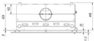
Wkład kominkowy MILA 16 kW
