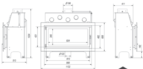
Wkład kominkowy MILA 16 kW
