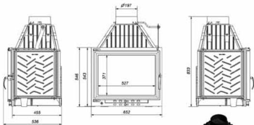
Wkład kominkowy ZUZIA EKO 16kW
