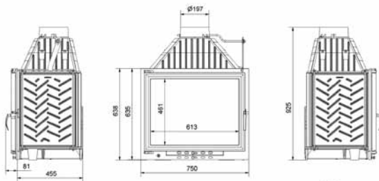
Wkład kominkowy AMELIA EKO 18 kW
